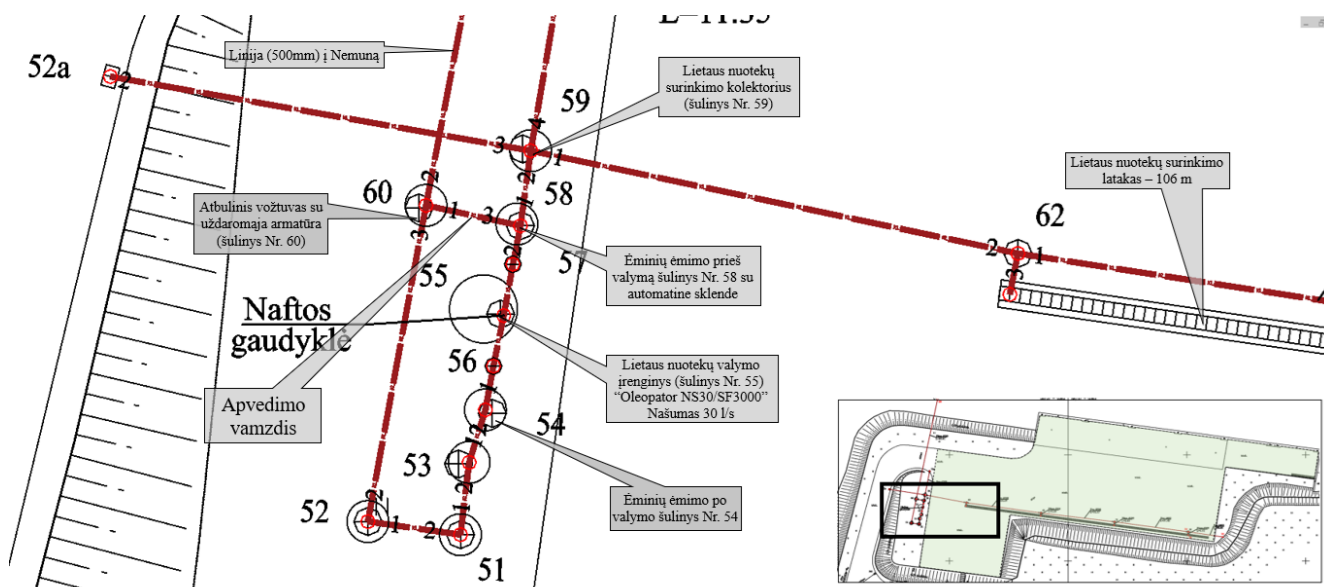
17 pav. Marvelės krovinės prieplaukos lietaus nuotekų tinklų su valymo įrenginiu schemas fragmentas (Šaltinis: žemės sklypo registro Nr. 44/1444214, Užnemunės g. 5, Kaunas, Kadastrinių matavimų byla / inžineriniai statiniai / nuotekų tinklai, žr. priede)
