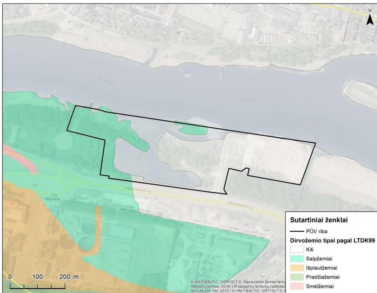
21 pav. Dirvožemio dangos tipai pagal LTK994
