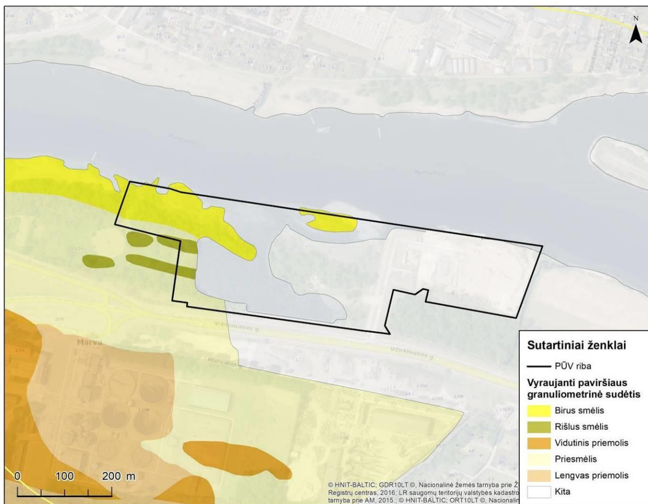
22 pav. Vyraujanti paviršiaus granulimetrinė sudėtis
