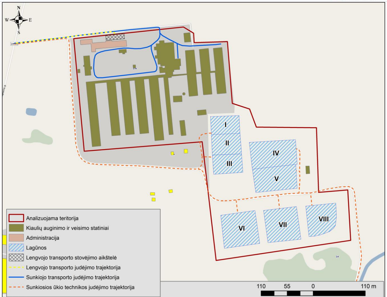
2 pav. Kiaulių auginimo komplekso situacijos schema
