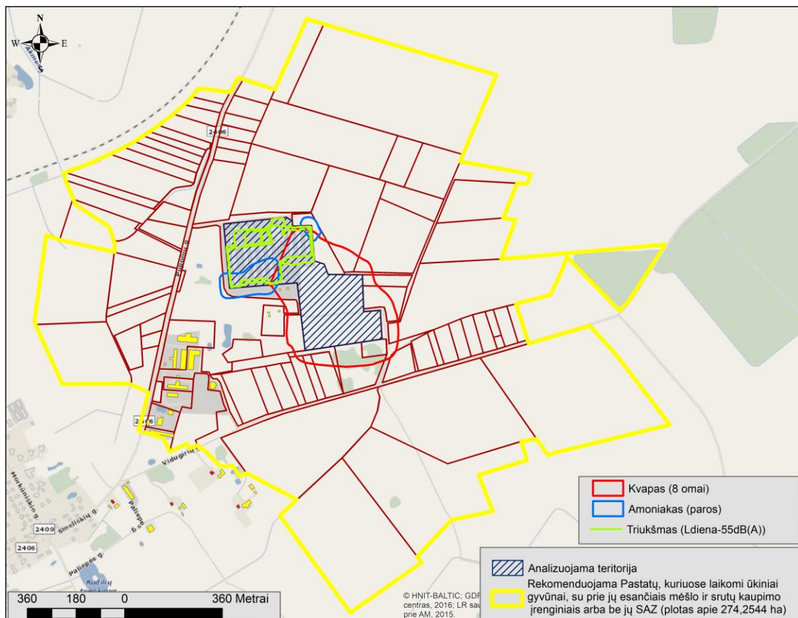
15 pav. Rekomenduojama „Pastatų, kuriuose laikomi ūkiniai gyvūnai, su esančiais prie jų mėšlo ir srutų kaupimo įrenginiais arba be jų, sanitarinė apsaugos zona“ su triukšmo, oro taršos ir kvapų viršnorminėmis izolinijomis tik nuo kiaulių auginimo veiklos
