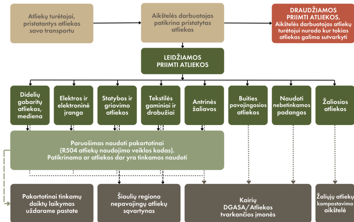
2 pav. Atliekų priėmimo ir tvarkymo principinė technologinė schema
