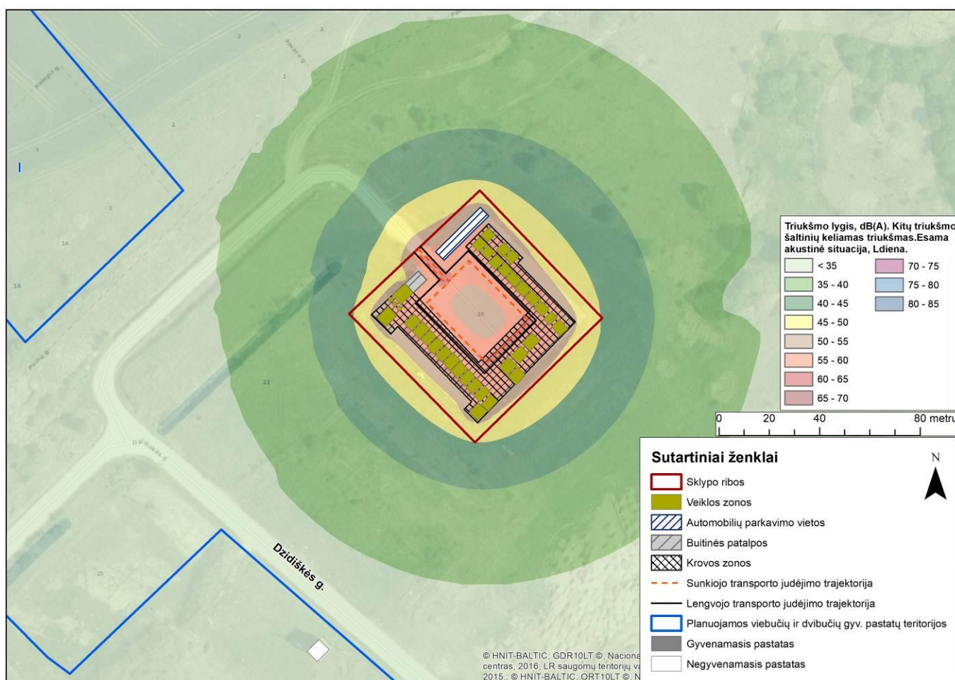
10 pav. Esamos akustinės situacijos triukšmo sklaida, kitų triukšmo šaltinių keliamas triukšmas, Ldiena
