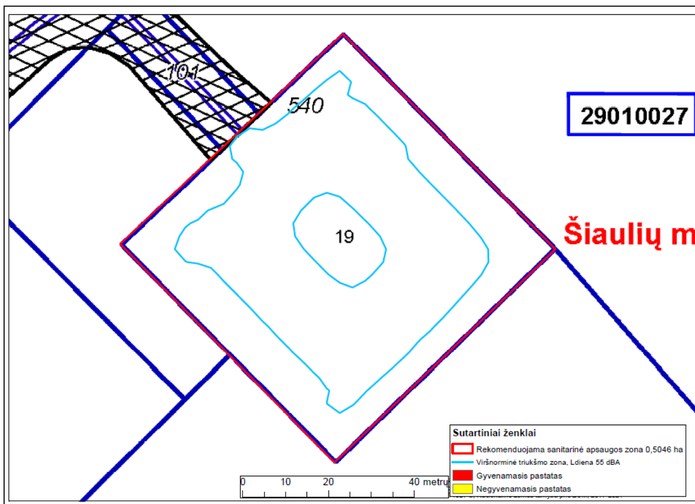
16 pav. Rekomenduojama sanitarinė apsaugos zona su triukšmo lygių viršijimo izolinijomis
