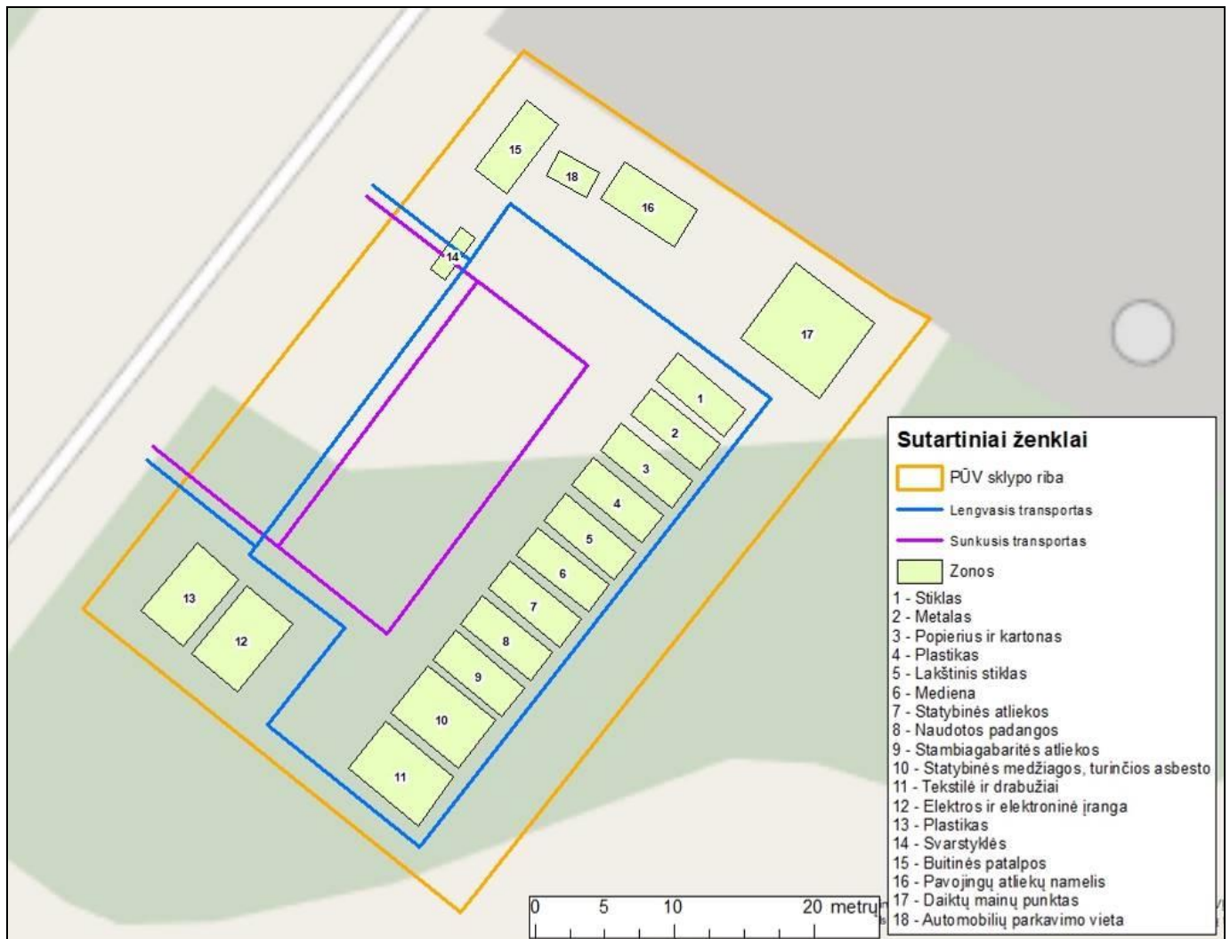
1 pav. Pakruojo (Kuosiškių k., Pakruojo sen., Pakruojo r. sav.) DGASA veiklos zonų išdėstymas
