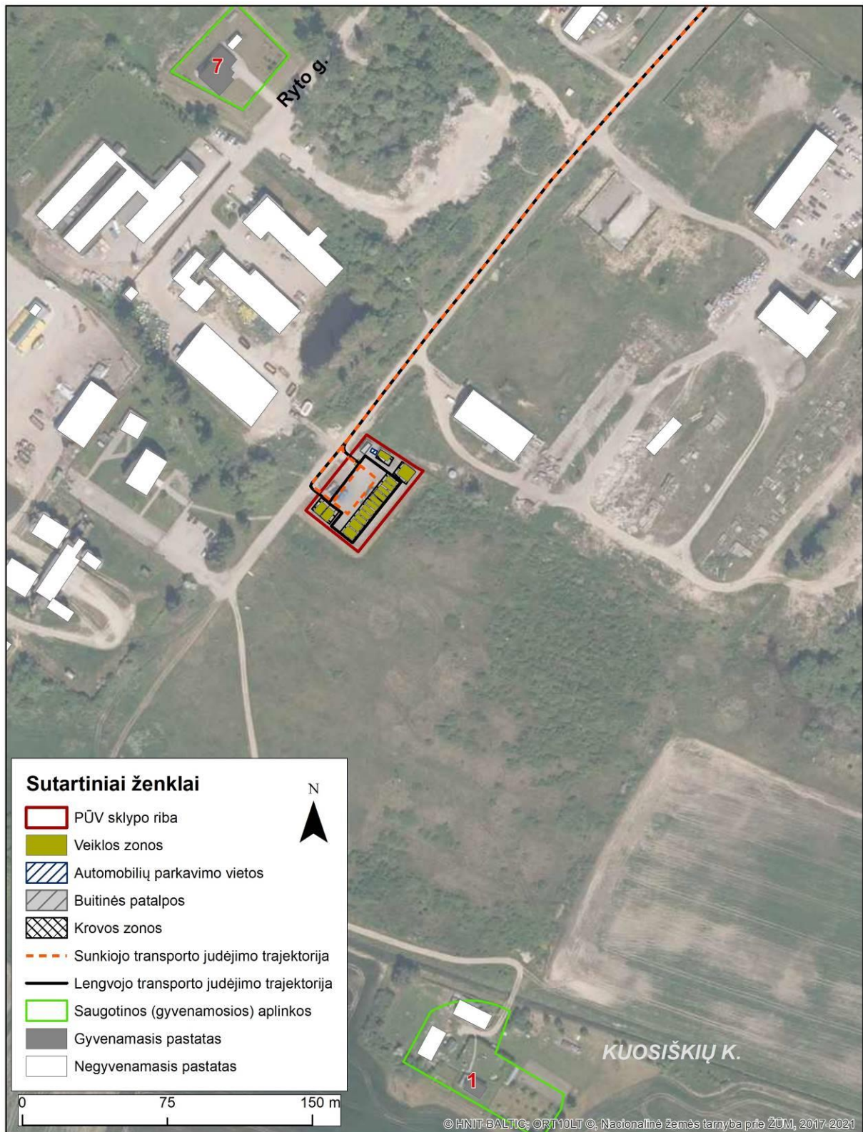
7 pav. Situacijos schema ir artimiausios saugotinos (gyvenamosios) aplinkos
