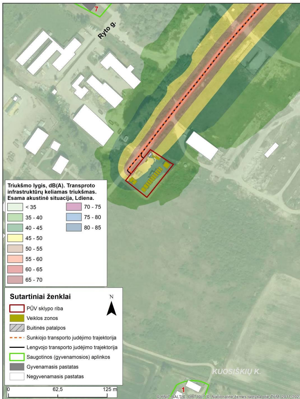
8 pav. Esamos akustinės situacijos triukšmo sklaida, transporto infrastruktūrų keliamas triukšmas, Ldiena
