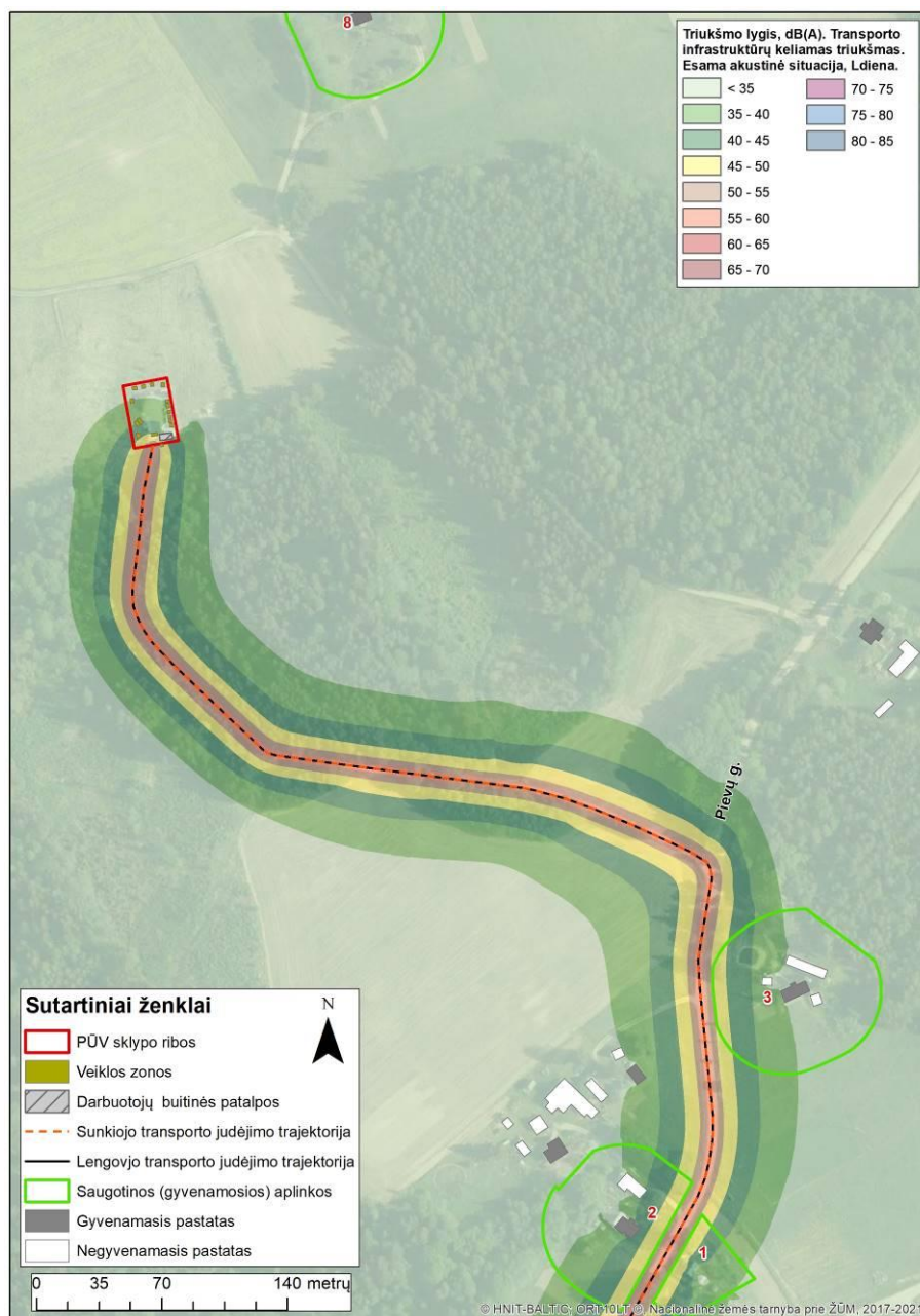
9 pav. Esamos akustinės situacijos triukšmo sklaida, transporto infrastruktūrų keliamas triukšmas, Ldiena
