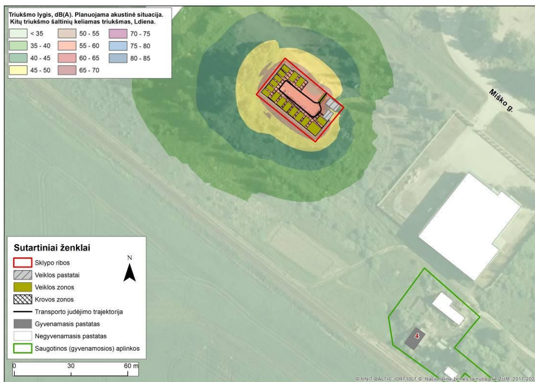
9 pav. Esamos akustinės situacijos triukšmo sklaida, kitų triukšmo šaltinių (ne transporto infrastruktūrų) keliamas triukšmas, Ldiena
