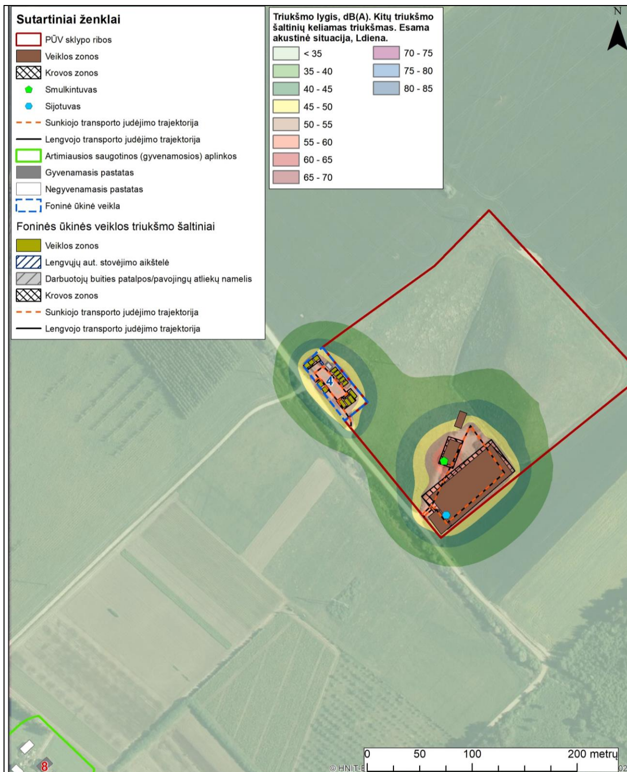
10 pav. Esamos akustinės situacijos triukšmo sklaida, suminis kitų triukšmo šaltinių (ne transporto infrastruktūrų) keliamas triukšmas, Ldiena
