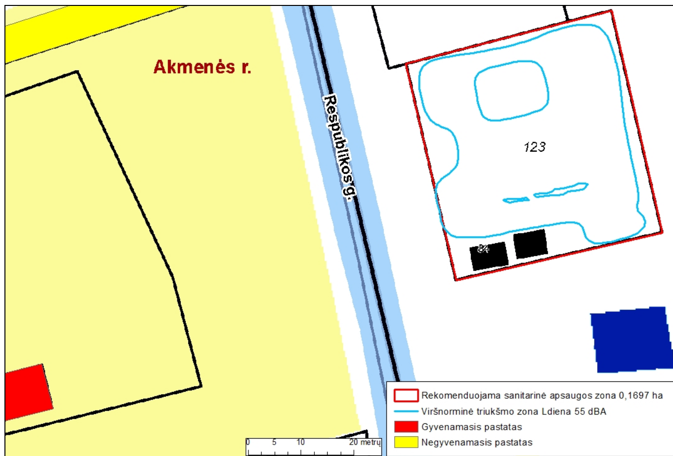
13 pav. Rekomenduojama sanitarinė apsaugos zona su triukšmo lygių viršijimo izolinijomis
