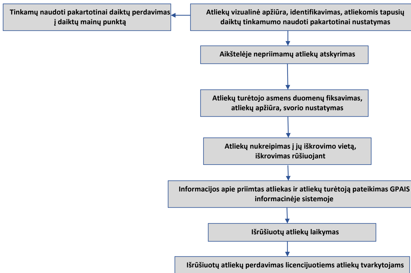
pav. Atliekų priėmimo ir tvarkymo principinė technologinė schema
