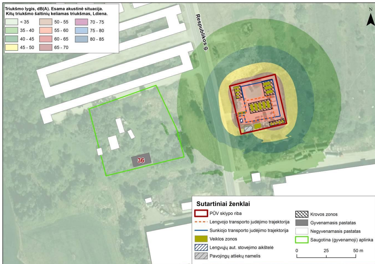
7 pav. Esamos akustinės situacijos triukšmo sklaida, kitų triukšmo šaltinių keliamas triukšmas, Ldiena
