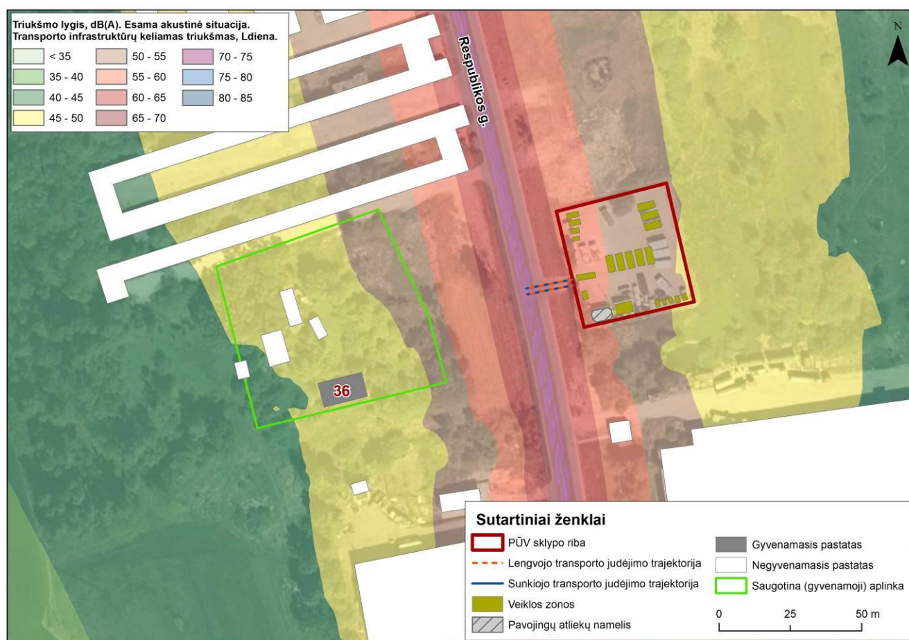
6 pav. Esamos akustinės situacijos triukšmo sklaida, transporto infrastruktūrų keliamas triukšmas, Ldiena
