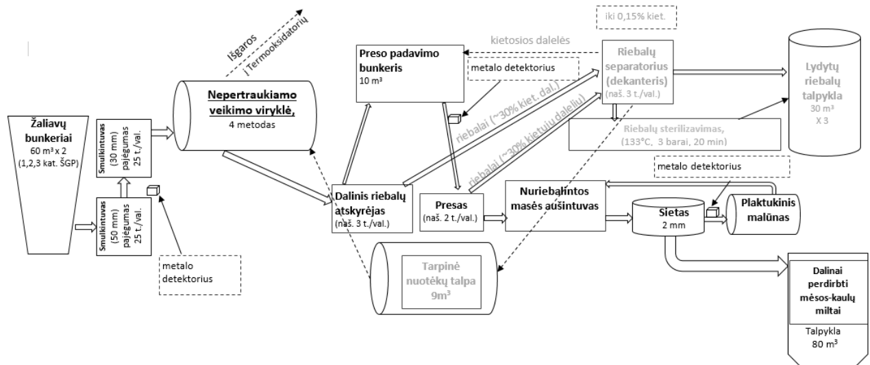
2 pav. 1 ir 2 kategorijos ŠGP tvarkymo padalinio perdirbimo linija
