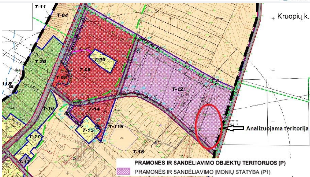
5 pav. Labūnavos kaimo detaliojo plano (patvirtintas 2014-06-19, įsakymo Nr. AD-1-790) pagrindinių sprendinių brėžinio ištrauka
