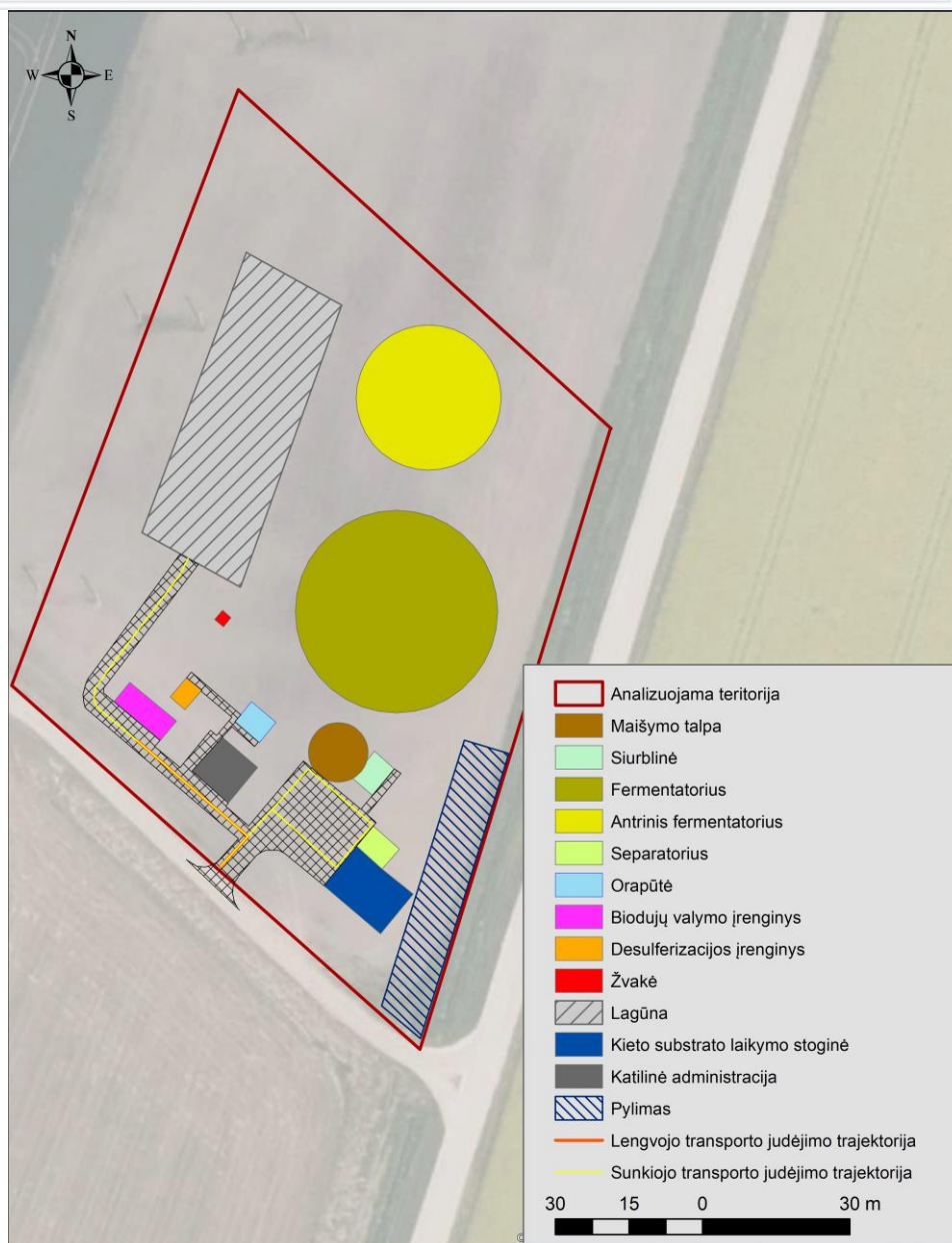
3 pav. Planuojamos biodujų jėgainės situacijos schema
