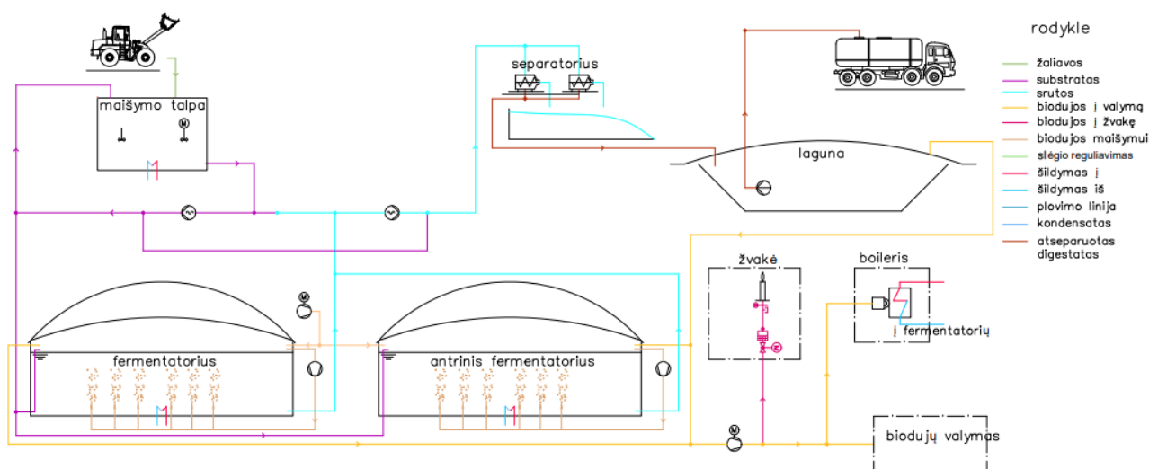
2 pav. Technologinė schema
