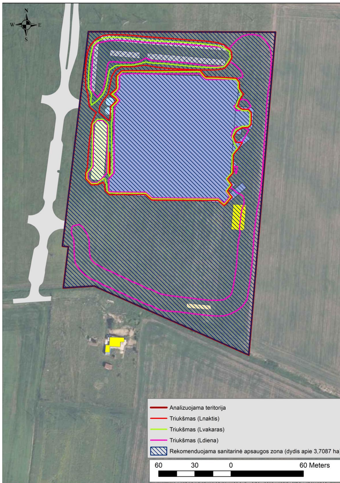
14 pav. Rekomenduojama sanitarinė apsaugos zona su triukšmo lygių viršijimo izolinijomis
