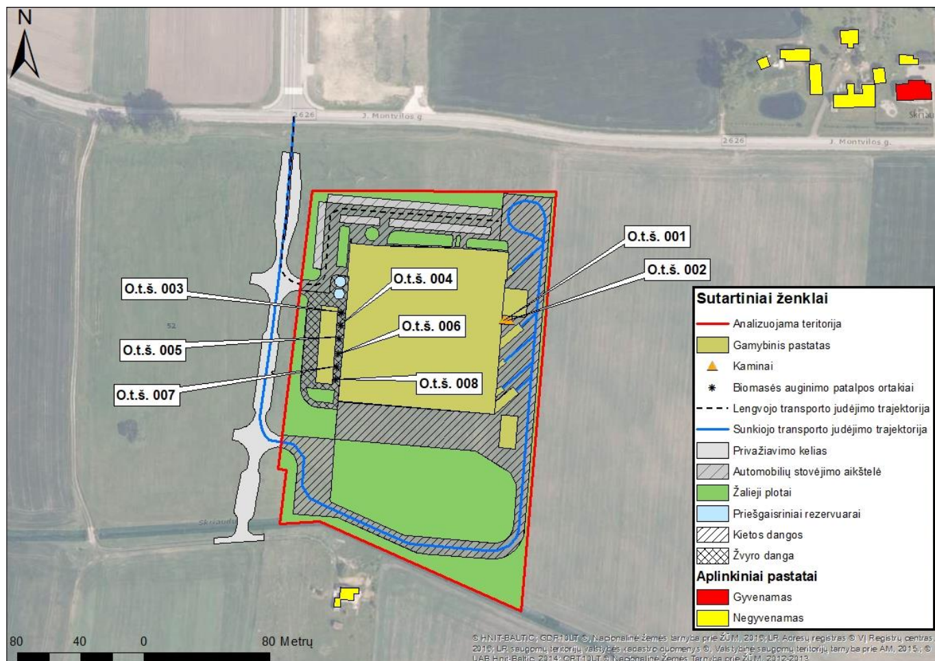
7 pav. Stacionarių oro taršos šaltinių išsidėstymo teritorijoje schema
