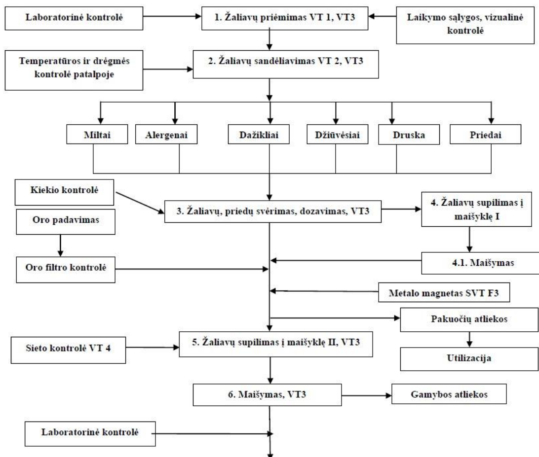
2 pav. Miltinių mišinių gamybos srauto diagrama
