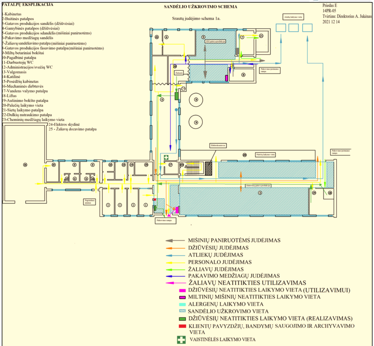
4 pav. UAB „Šlaituva“ džiovėsių ir miltinių mišinių gamybos įmonės vidaus patalpų schema
