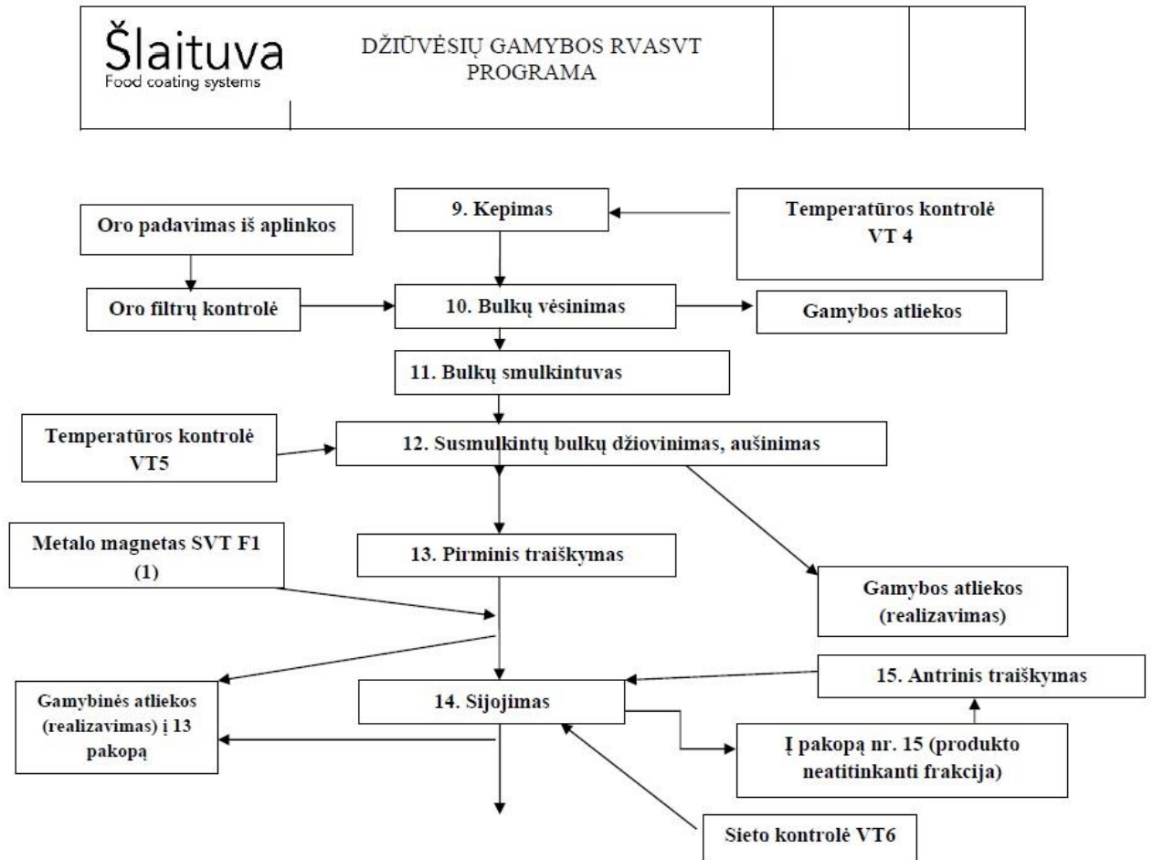
1 pav. Džiuvėsėlių gamybos sruto diagrama
