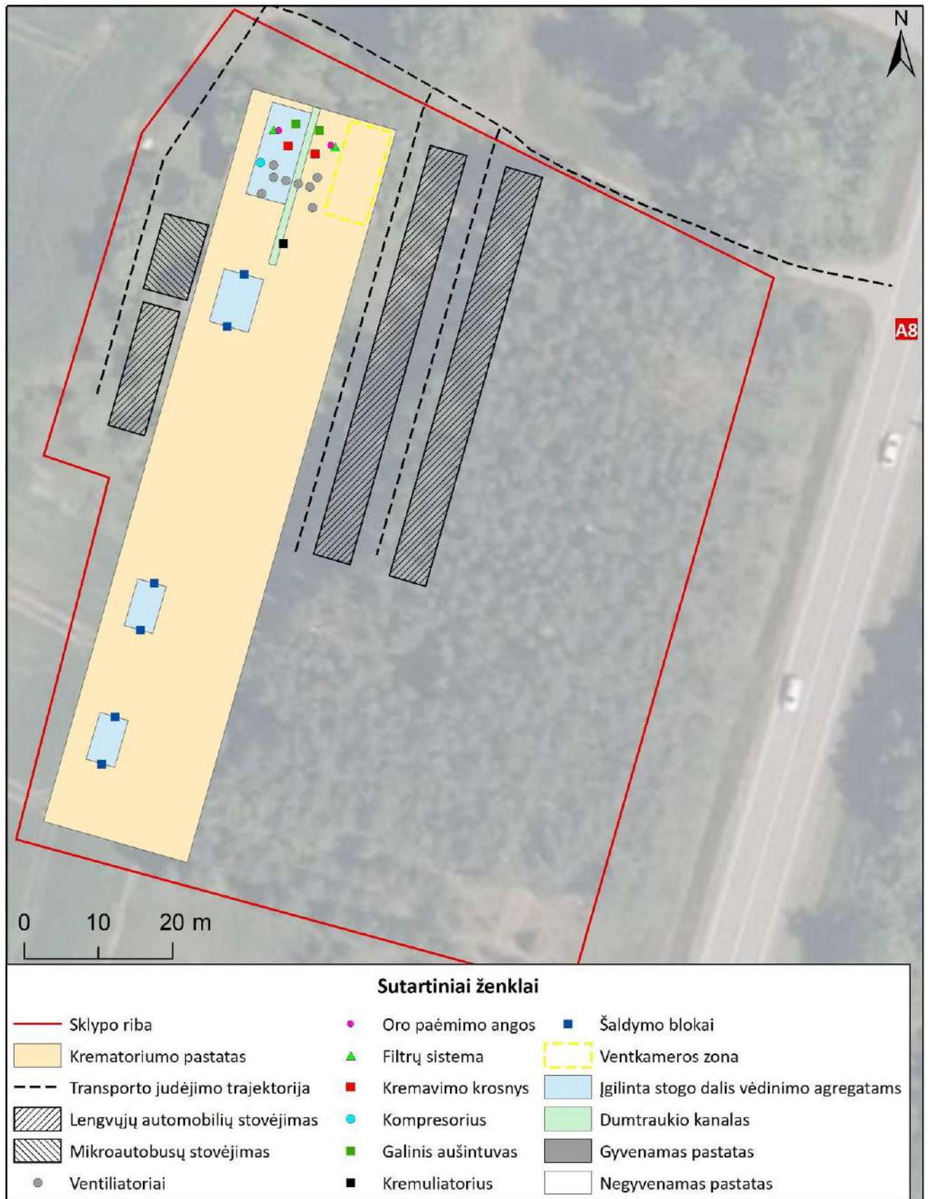
7 pav. PŪV planuojamų triukšmo šaltinių situacijos schema
