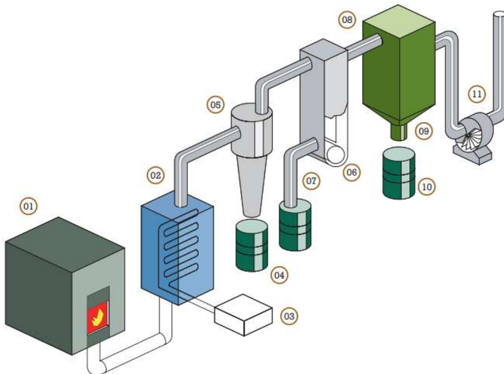
1 pav. Kremavimo įrangos išeinančių dūmų valymo sistema 3
