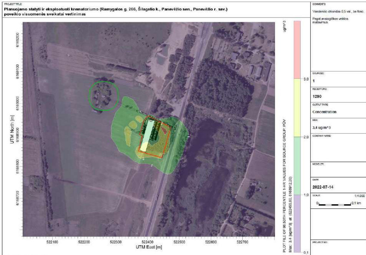
5 pav. Vandenilio chlorido pusės valandos sklaida
