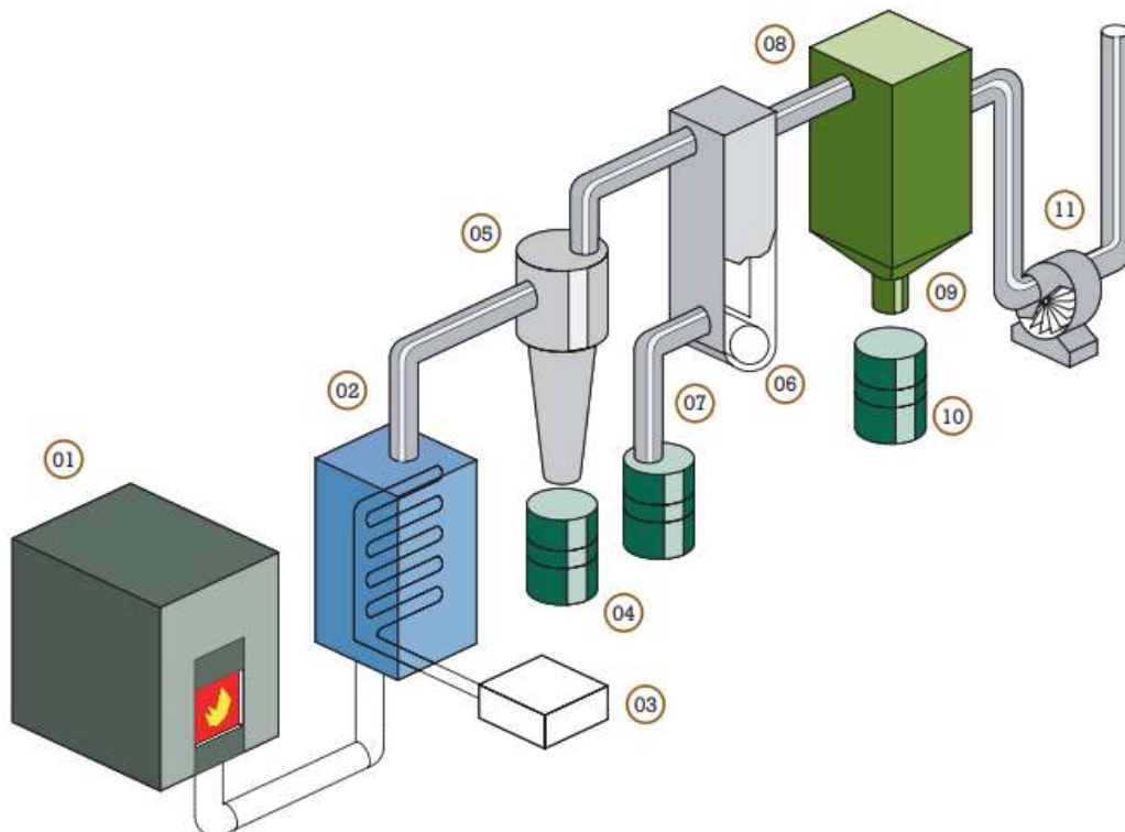
1 pav. Kremavimo įrangos išeinančių dūmų valymo sistema 3
