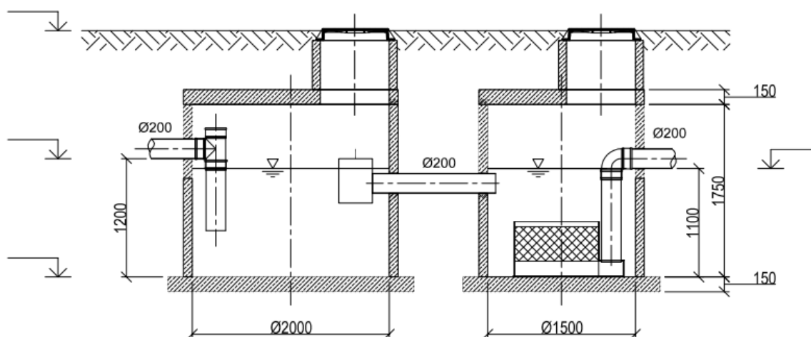
8 pav. Paviršinių nuotekų valymo įrenginio Tera δ-10 schema
