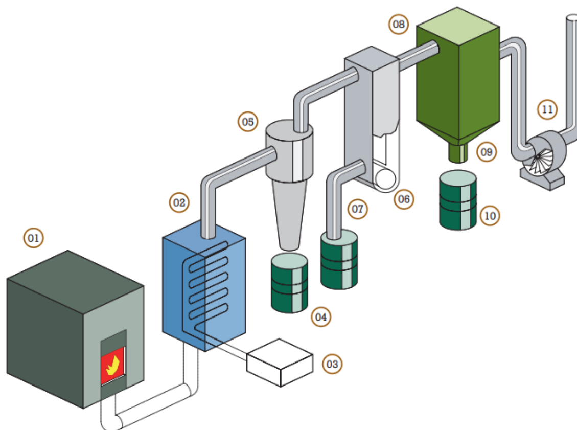
1 pav. Kremavimo įrangos išeinančių dūmų valymo sistema 1
