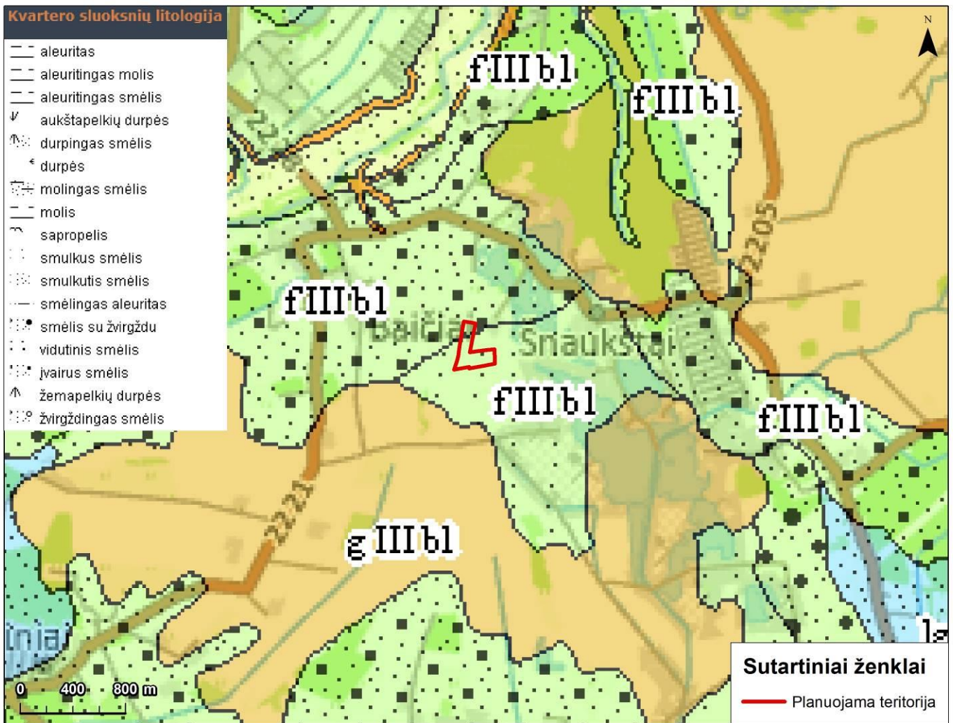
9 pav. Ištrauka iš kvartero geologinio žemėlapiu (www.lgt.lt)
