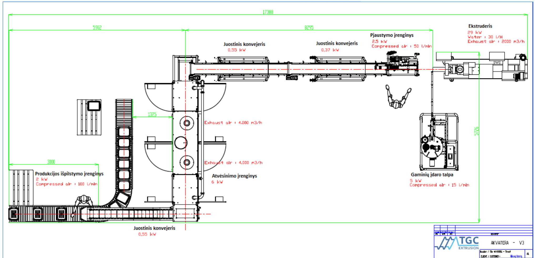
7 pav. Skanėstų šunims ir katėms ko-ekstruzijos būdu (pagalvėlės su įdaru), gamybos linijos techninės schema
