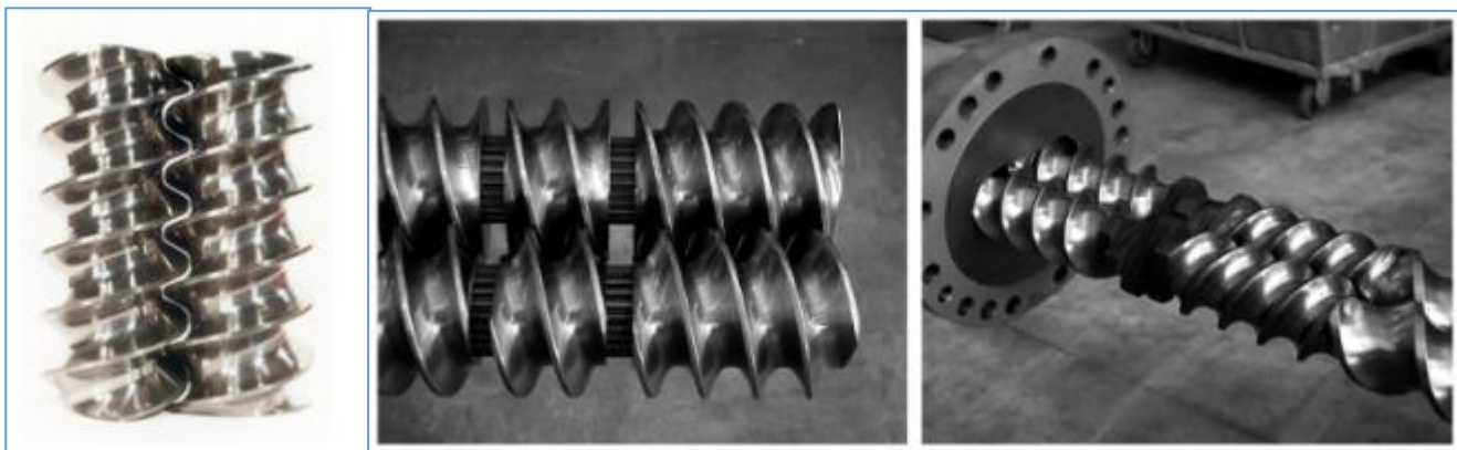
2 pav. Du ant velenų besisukantys sraigtai, montuojami ekstruderio korpuso viduje („Cletral“, „Pavan Group“)
