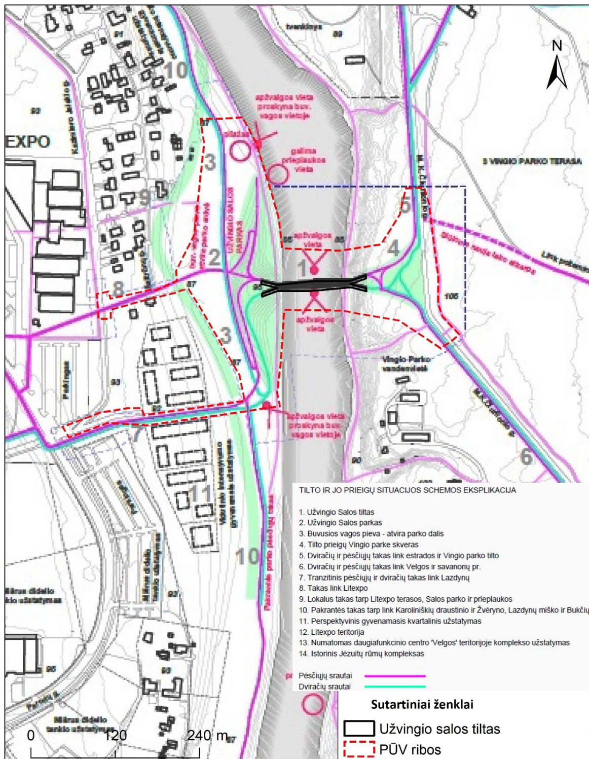
6. pav. Detaliojo plano ribose, inžinerinės infrastruktūros koridoriaus zonoje planuojamo tilto su pėsčiųjų ir dviračių takais situacijos schema
