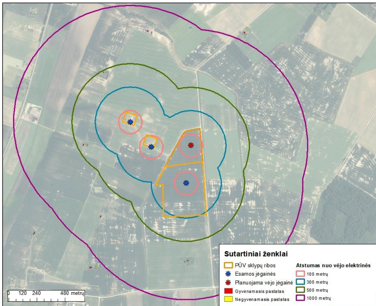
15 pav. VE vietos bei 1 km atstumu esantys pastatai
