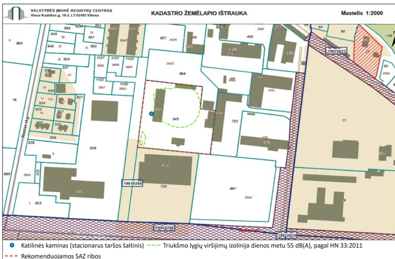
14 pav. Triukšmo lygių viršijimų izolinijos ir rekomenduojamos SAZ ribos
