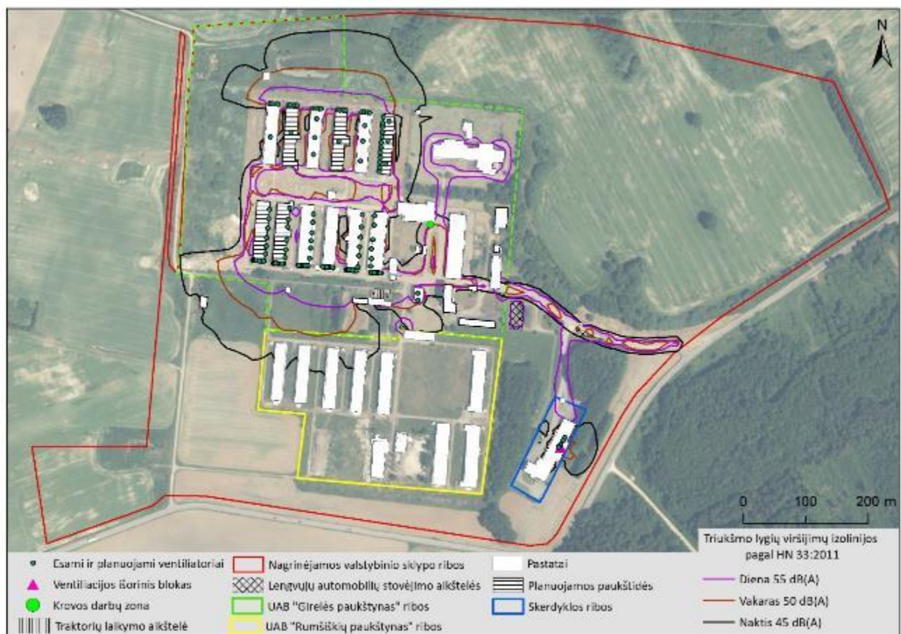
58 pav. Sumodeliuotas projektinės situacijos triukšmo ribinių verčių viršijimo izolinijos analizuojamoje teritorijoje, be foninių triukšmo šaltinių
