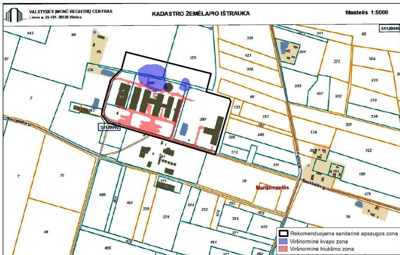
21 pav. Kvapo ir triukšmo ribinių dydžių viršijimo zona ir rekomenduojama sanitarinė apsaugos zona
