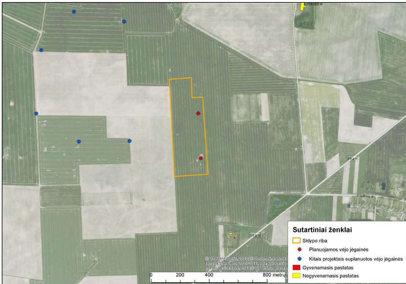
1 pav. Planuojama statyti ir kitais projektais numatytos vėjo elektrinės, jų padėtytys
