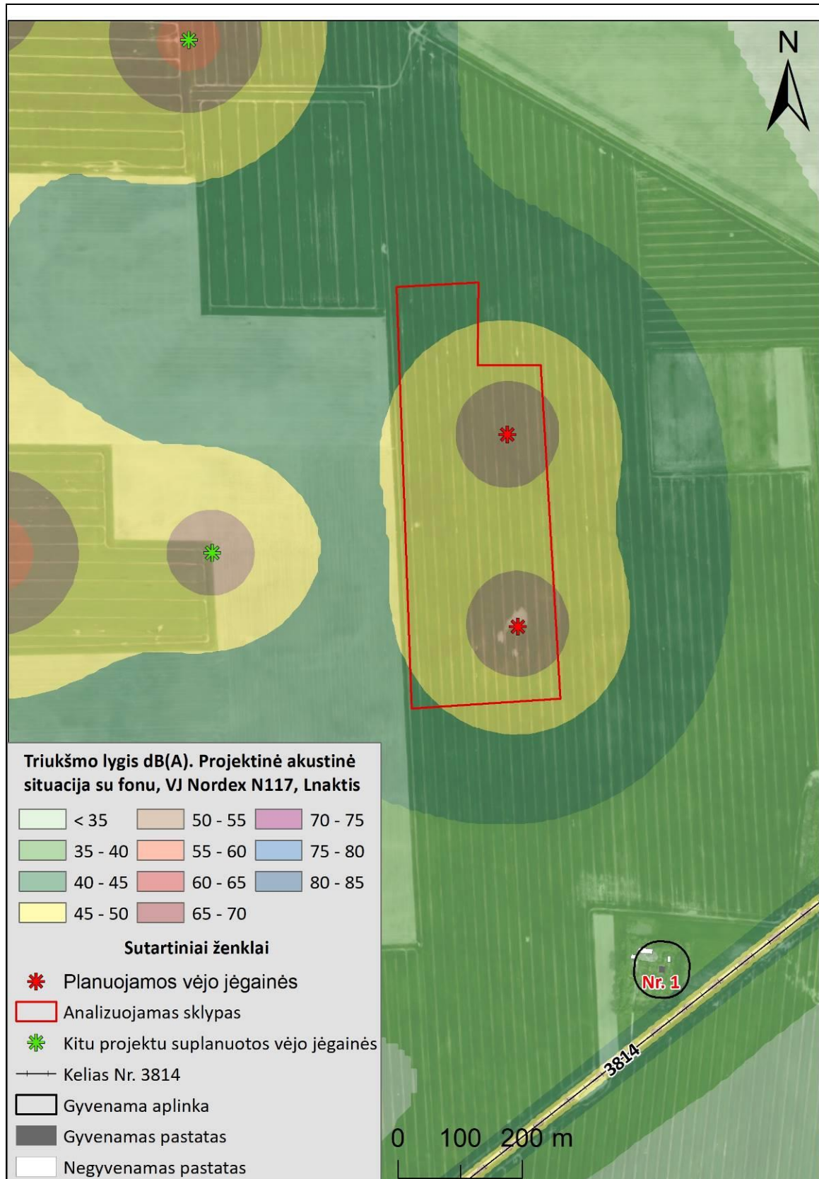
15 pav. Triukšmo sklaida nakties metu su fonu (L nakties), VJ modelis Nordex N117
