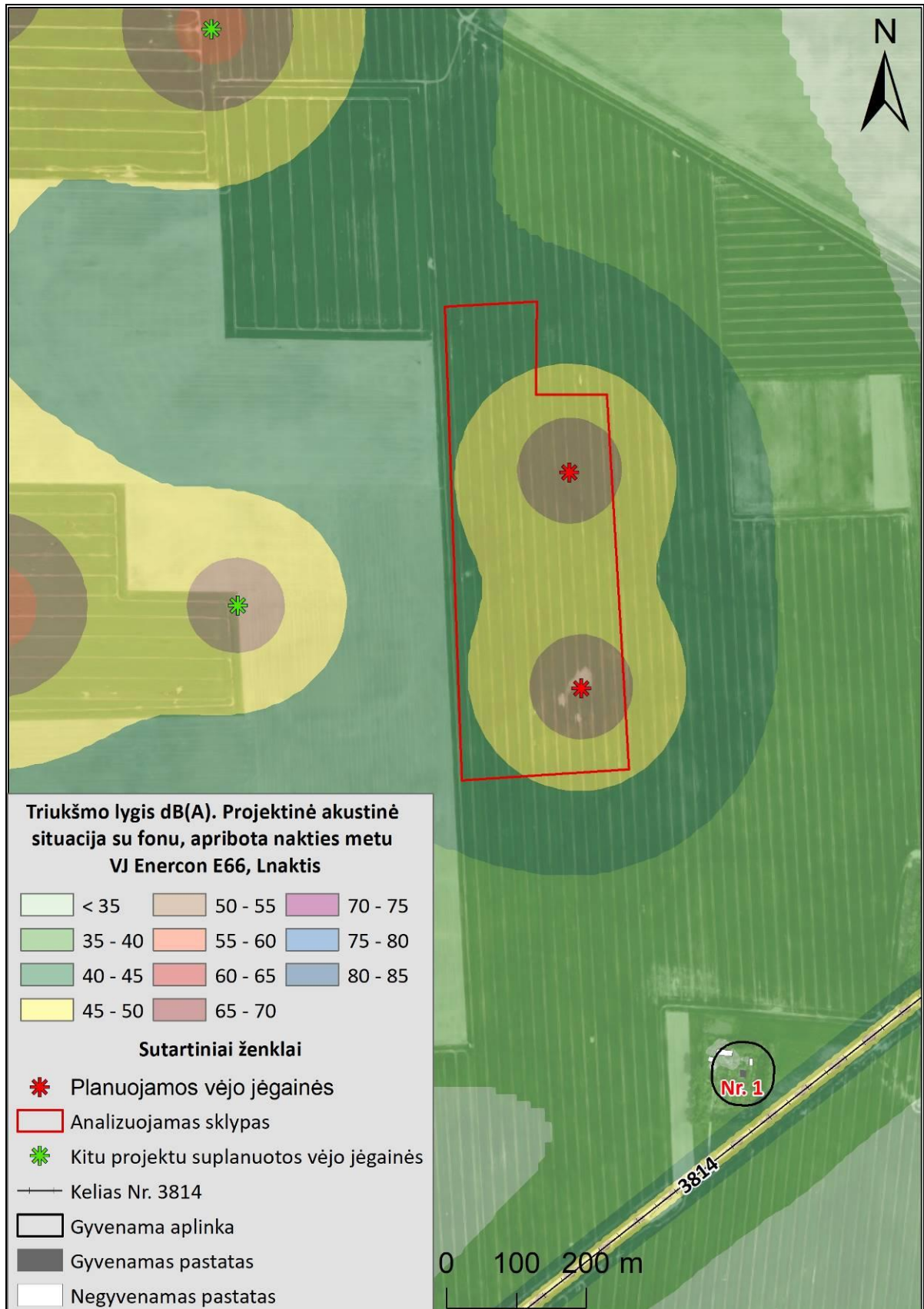
14 pav. Triukšmo sklaida nakties metu su fonu (L nakties), VJ modelis Enercon E66 apribotas nakties metu
