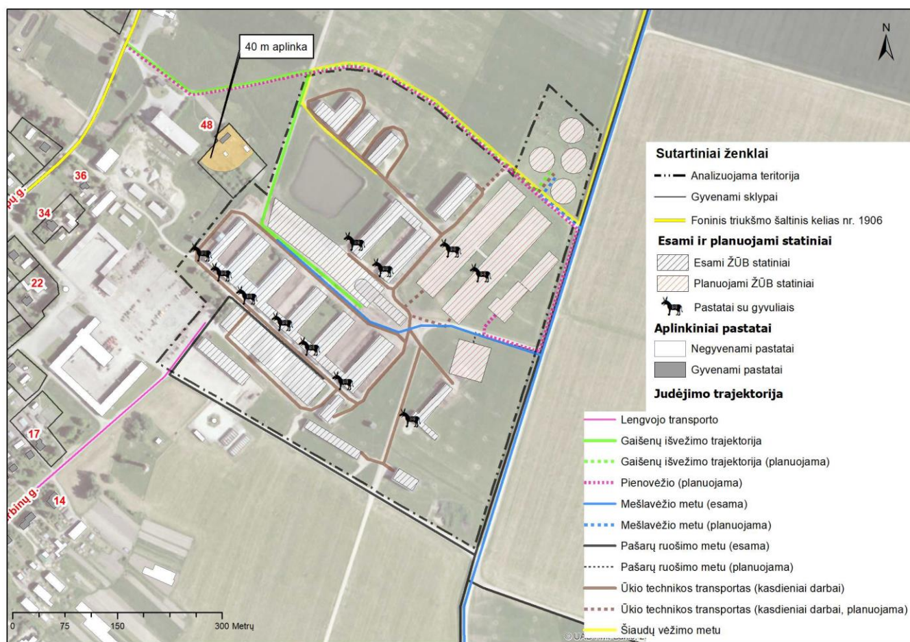
10 pav. Transporto judėjimo trajektorijos ir artimiausias gyvenamas pastatas
