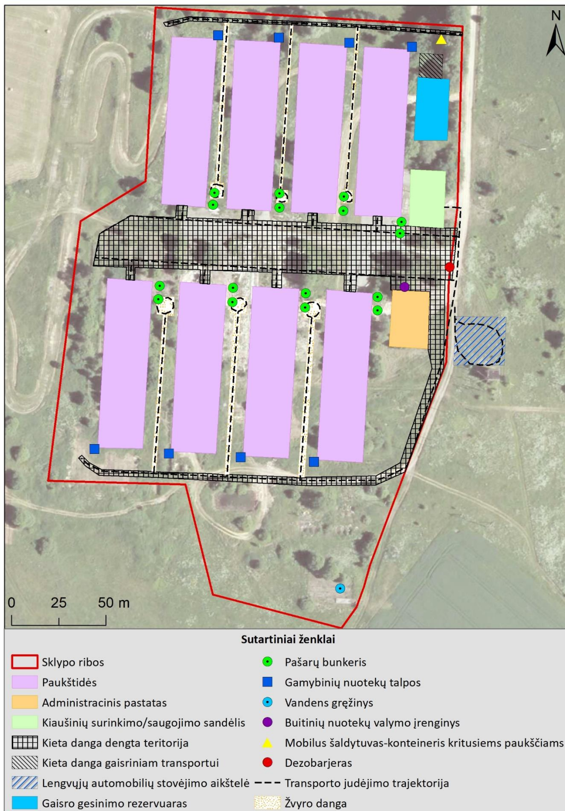
4 pav. Planuojamų statinių, įrenginių, aikštelių išsidėstymo schema
