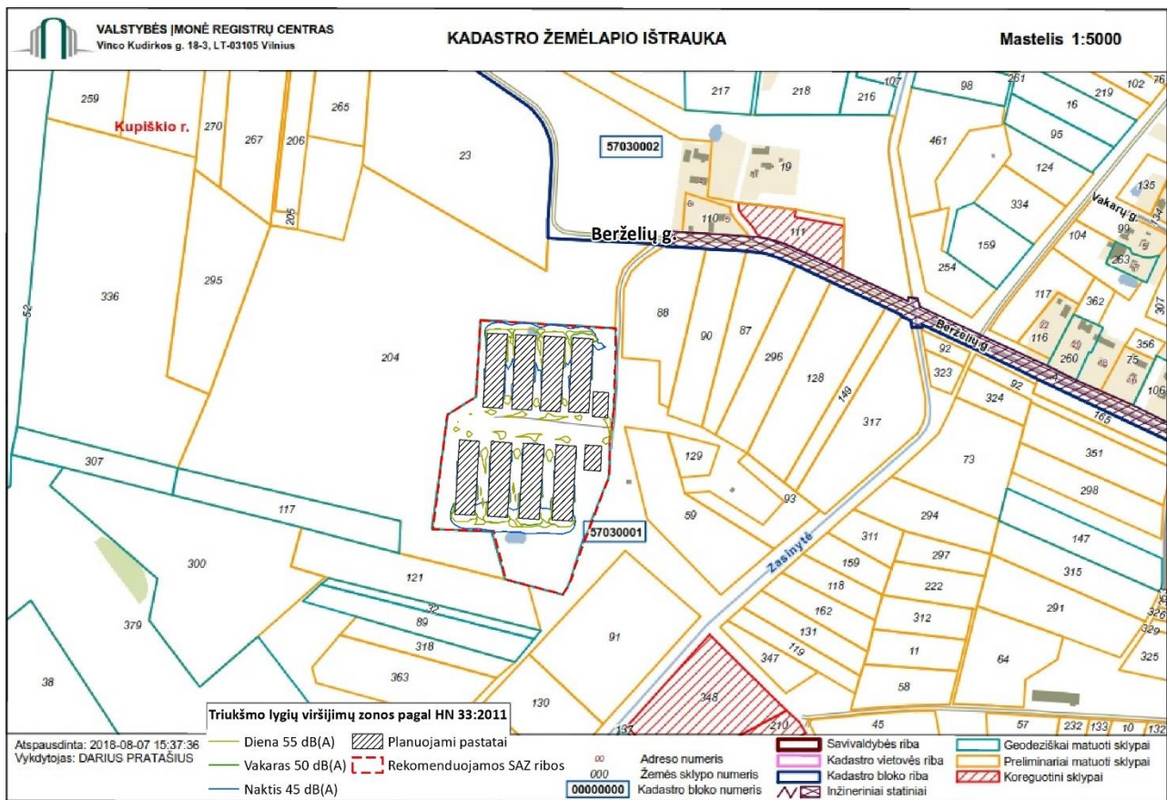
38 pav. Triukšmo lygių izolinijos ir rekomenduojama SAZ
