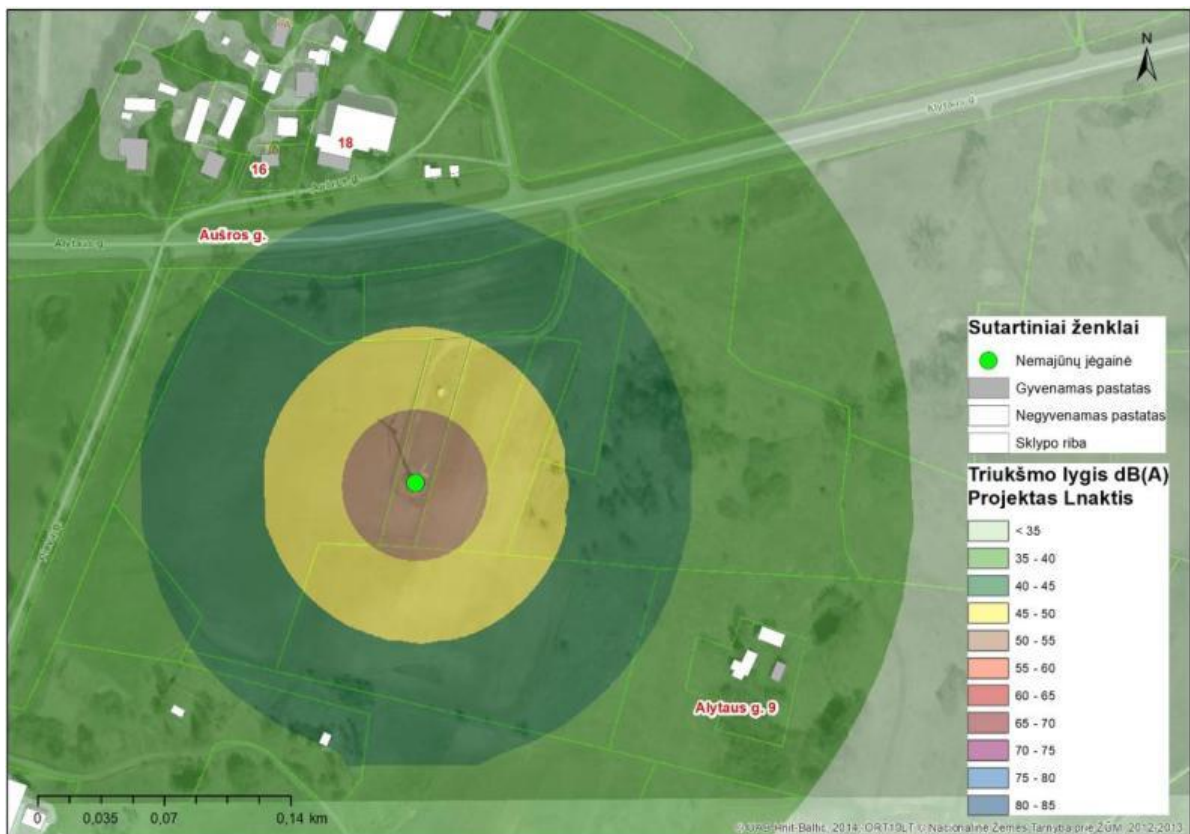
13 pav. Triukšmo sklaida be fono nakties metu (L nakties)
