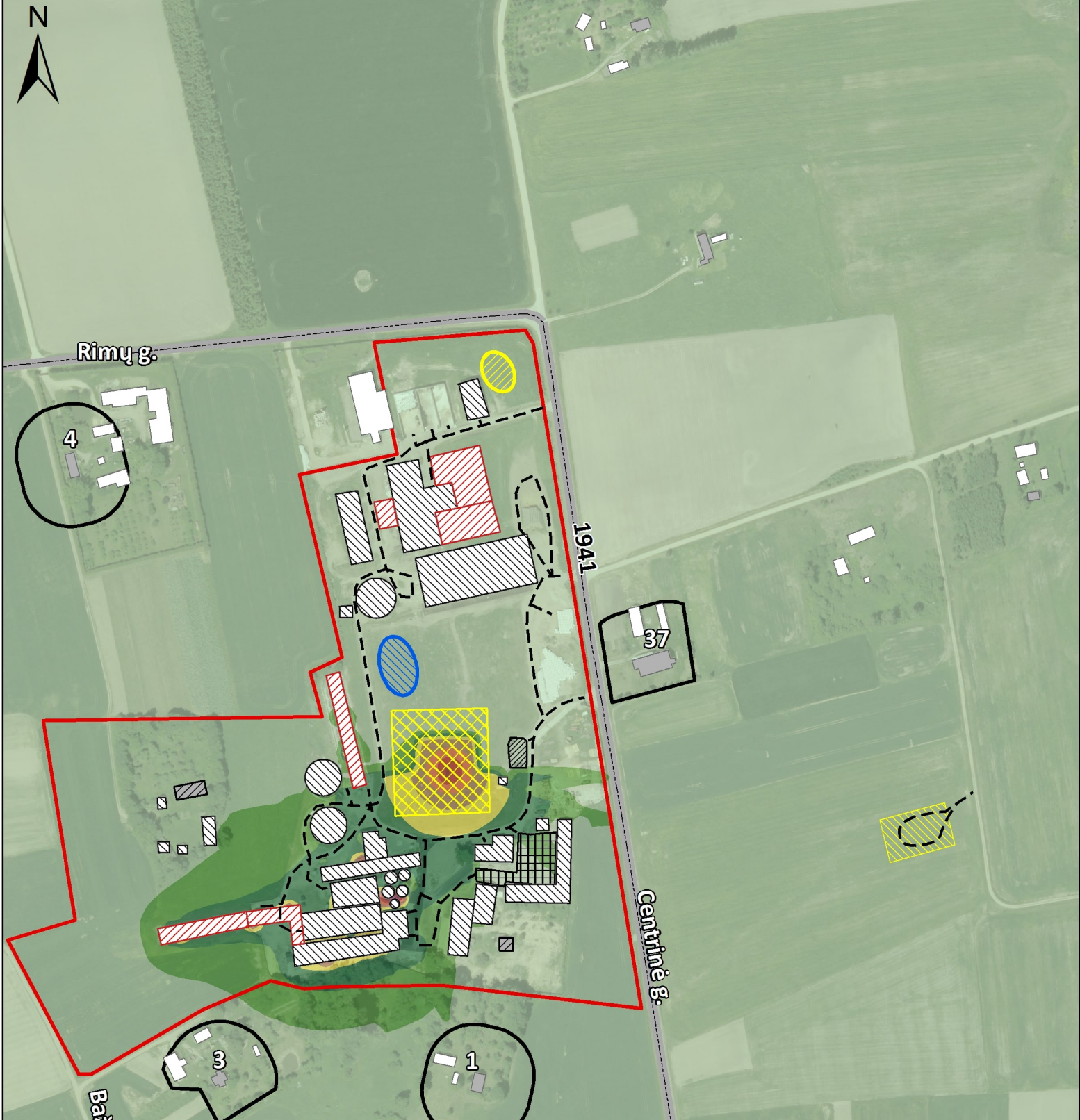
Triukšmo lygis dB(A). Projektinė situacija be fono, Lvakaras
