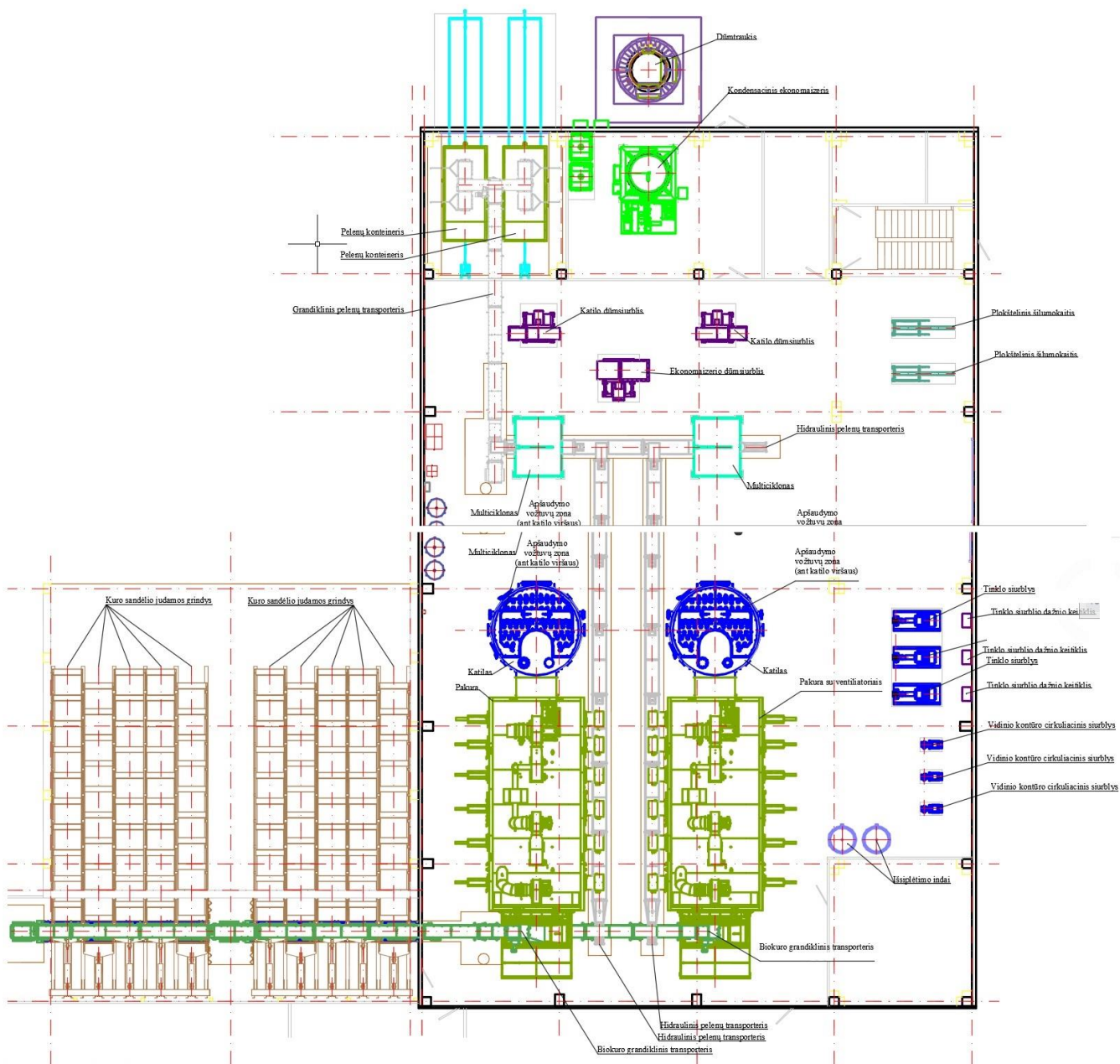
8 pav. Įrenginių išdėstymo planas
