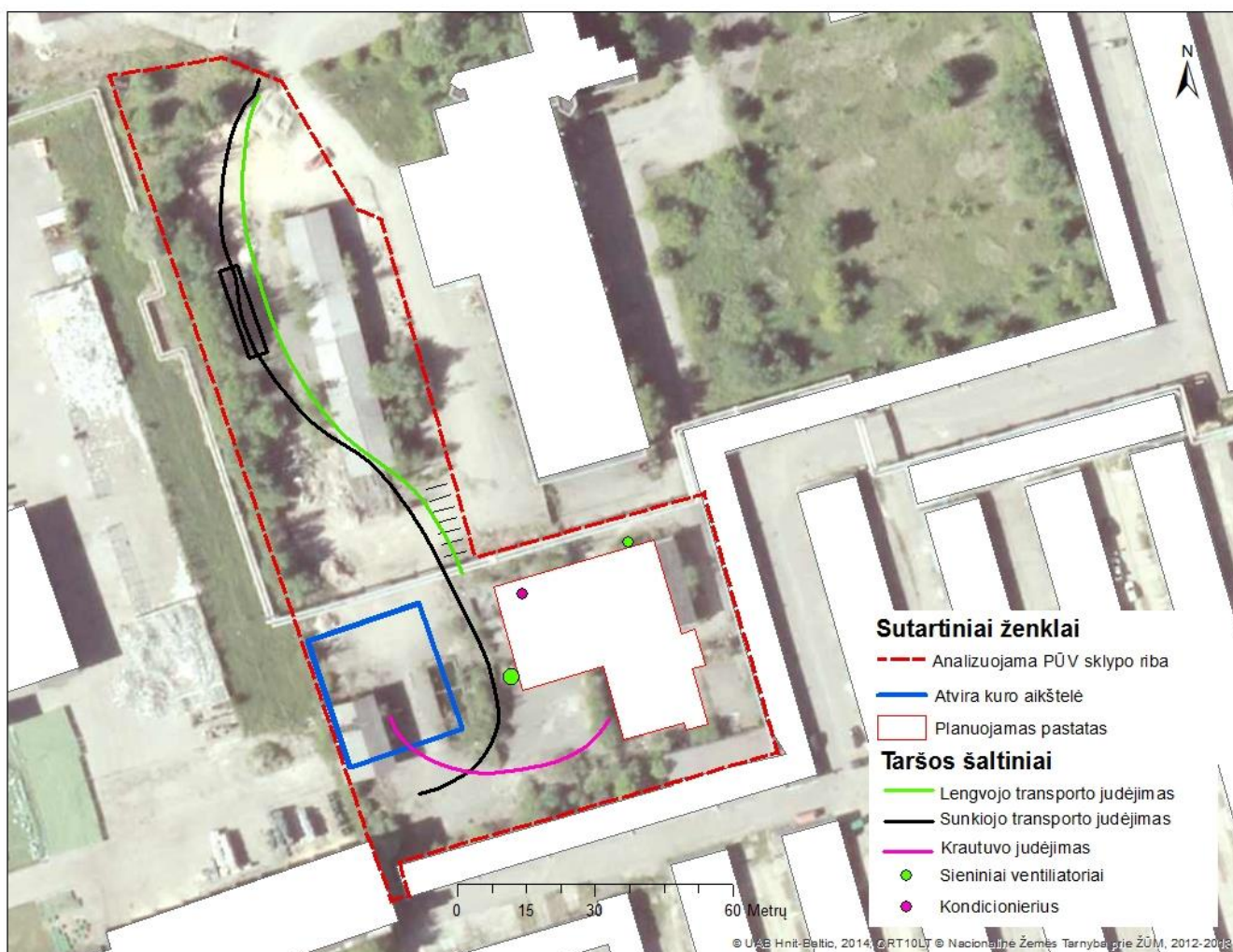
9 pav. Planuojamos situacijos planas
